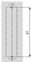
Rys. 5. Rozmieszczenie otworów w przypadku montażu na ścianie lub w płycie montażowej.
